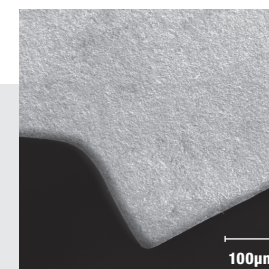
Schneidekante und Oberfläche nach dem Strahlen Cutting edge and surface after blasting 喷砂后刀片的切削刃和表面
